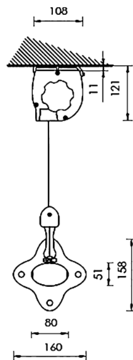
Montaje frontal
